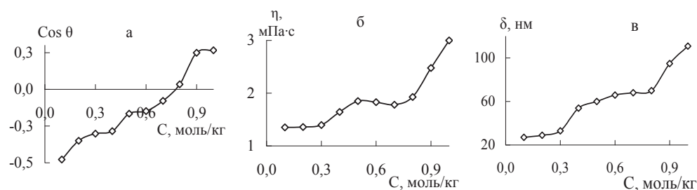
Рис. 2. Влияние концентрации (С) твердых растворов ФОР в парафине на: а – краевой угол смачивания ( \cos \theta ) их поверхности дистиллированной водой; б – динамическую вязкость ( \eta ) суспензий; в – толщину гидратной оболочки ( \delta ) частиц дисперсной фазы суспензий.
