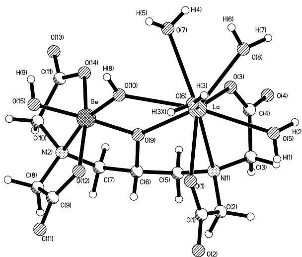
Рис. 3. Кристаллическая структура комплексной молекулы [\text{Ge}(\text{OH})(\mu\text{-Hpda})(\mu\text{-OH})\text{La}(\text{H}_2\text{O})_4]
