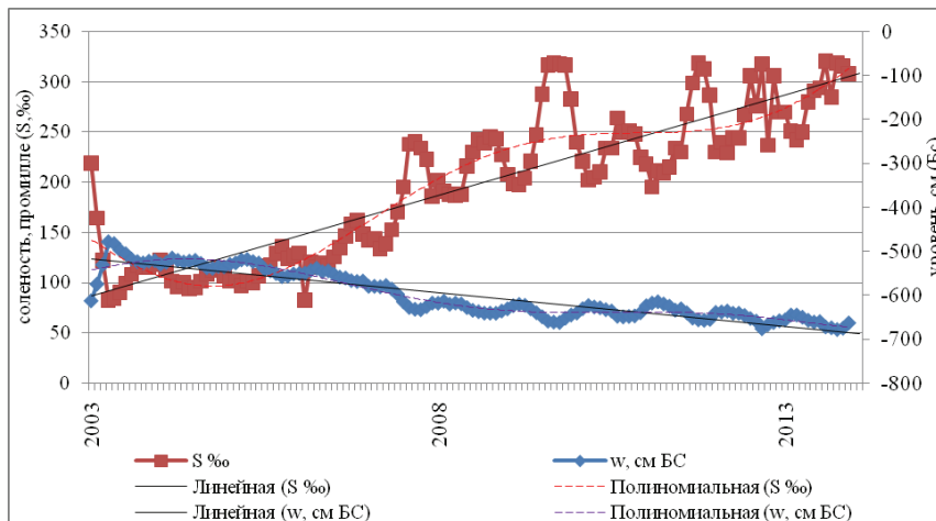
Рис. 3. Среднемесячная динамика изменения солёности и уровня воды Кл в 2003-2013 гг.
