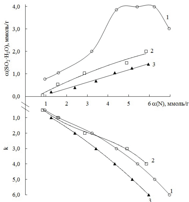
Рис. 3. Зависимость статической поглотительной емкости по SO 2 ( \alpha(SO_2 \cdot H_2O) , ммоль/г) и стехиометрического соотношения ( k ) образцов ИВХС–Ni–EDA (1), ИВХС–Ni–MEA (2) [27] и ИВХС–Cu–PEPA (3) [28] от содержания азота ( \alpha(N) , ммоль/г).
