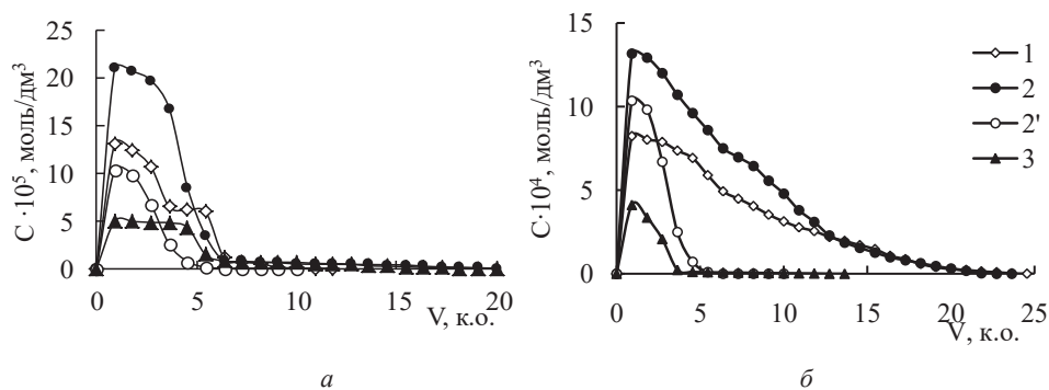
Рис. 4. Вихідні криві елювання урану з фази волокнистих іонітів ФІБАН К-1 (1), ФІБАН АК-22В (2, 2'), ФІБАН А-6 (3) 0,5 М розчинами НСl (1, 2, 3) або Н 2 SO 4 (2') після сорбції урану (VI) з сульфатних розчинів з рН 2 (1, 2, 3) та 4 (2').
