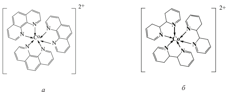
Рис. 3. Схеми будови комплексних катіонів в І ( a ), ІІ ( б )
